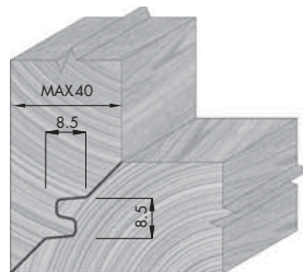
5.467 Gehrungs-Verleimfräser Porte-outils à bouquetage 45°
